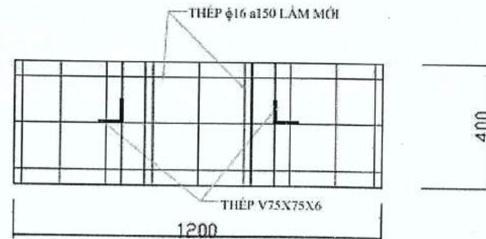
MẶT BẰNG MÓNG
