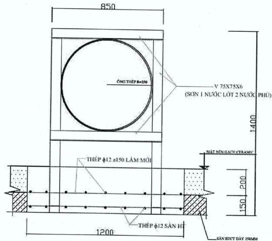
MẶT CẮT
