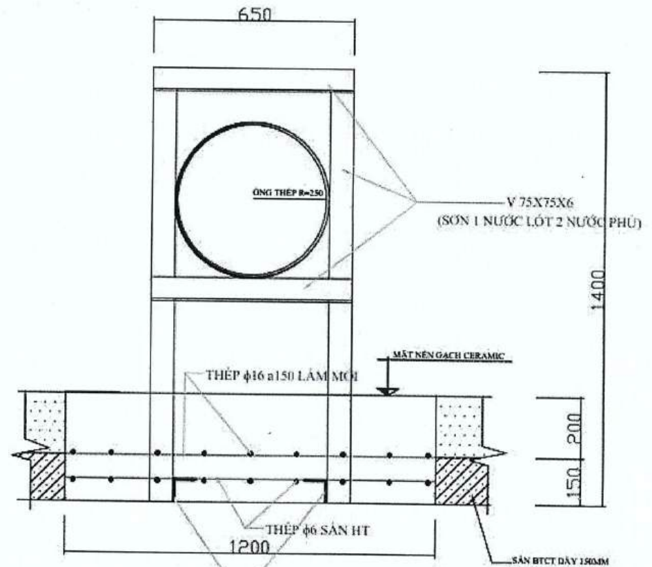
MẶT CẮT
